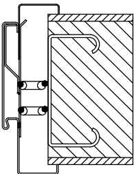
可调节框 VarioFrame 预埋件焊接 D1 型
