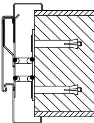
可调节框 VarioFrame 外加预埋件焊接 D2 型
